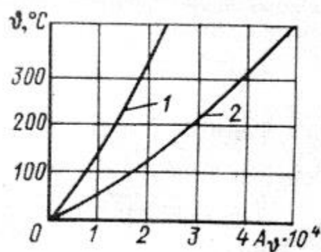
Рисунок 2 – Кривые для определения температуры нагрева токопроводов (1 - для алюминия, 2 - для меди)
