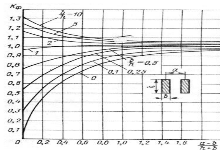
Рисунок 1 – Кривые для определения коэффициента формы K_{\phi}
